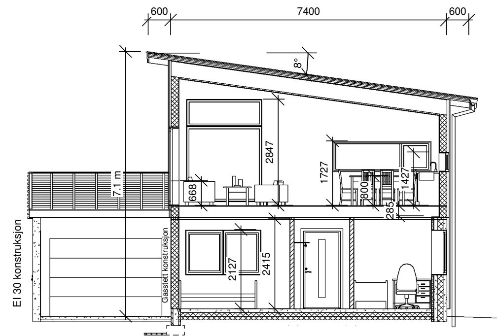
Snitt B 1 : 100
