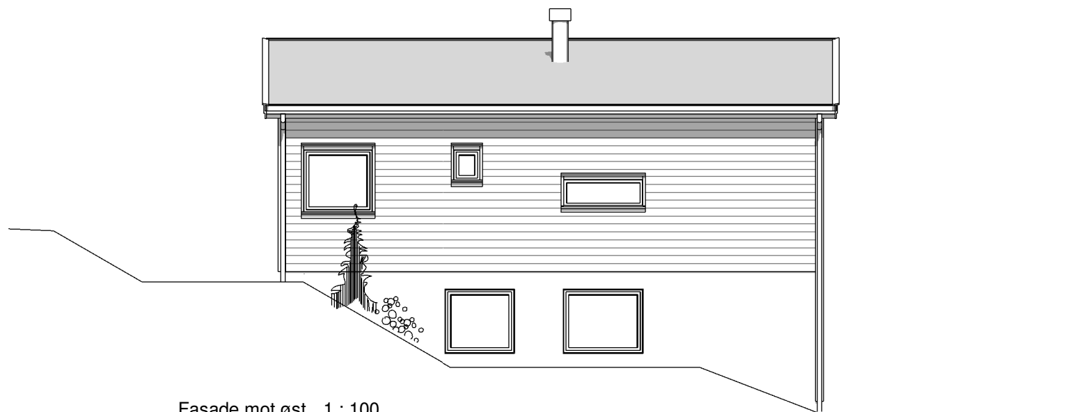
Fasade mot øst 1 : 100
