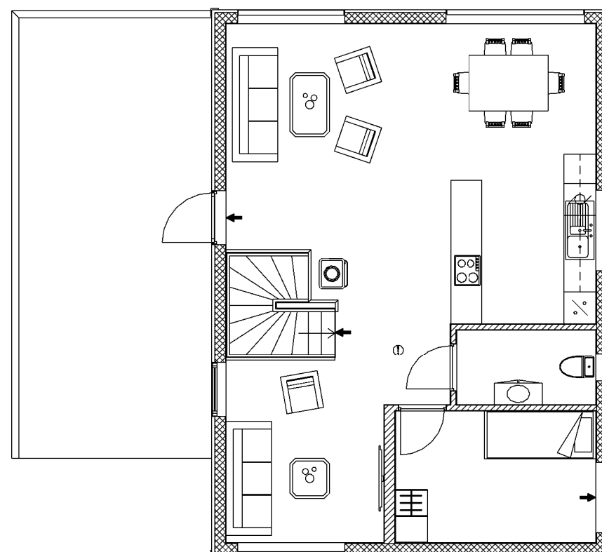
1.0 - 1.etasje plan 1 : 100
