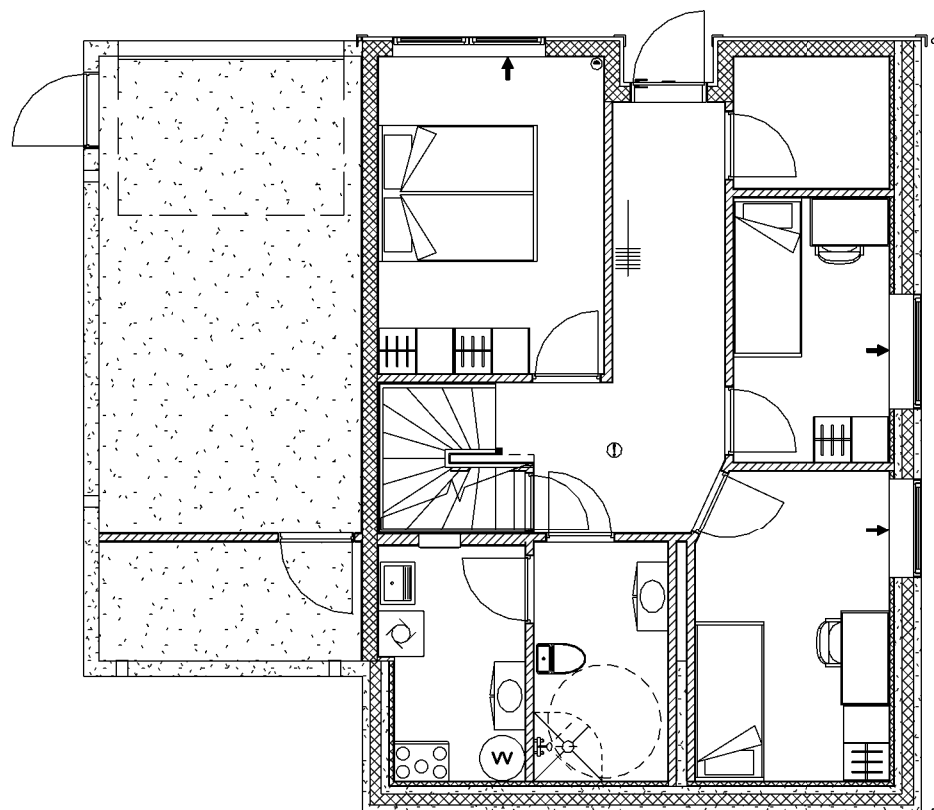
0.1 - Underetasje plan 1 : 100
