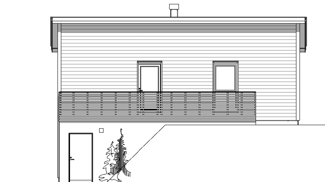
Fasade mot vest 1 : 100
