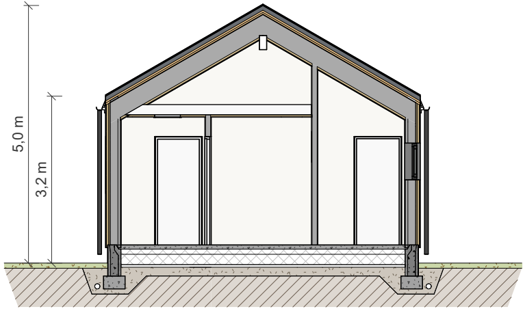
Snitt B1
