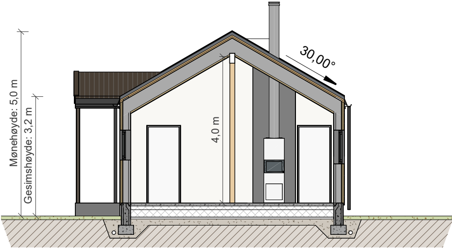
Snitt A1
