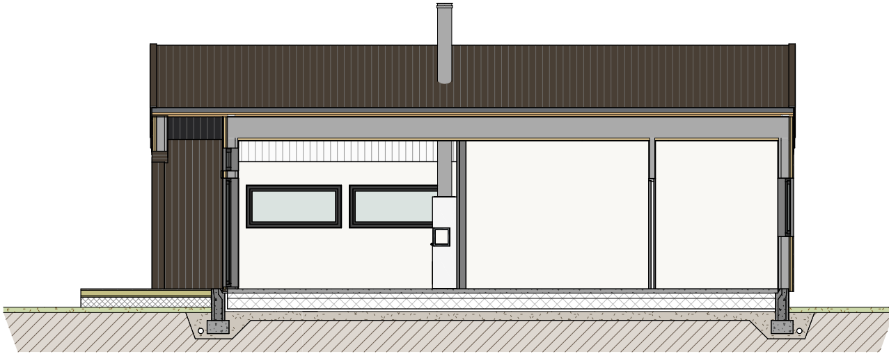
Snitt C1
